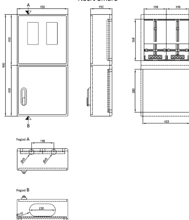
Načrt omare
