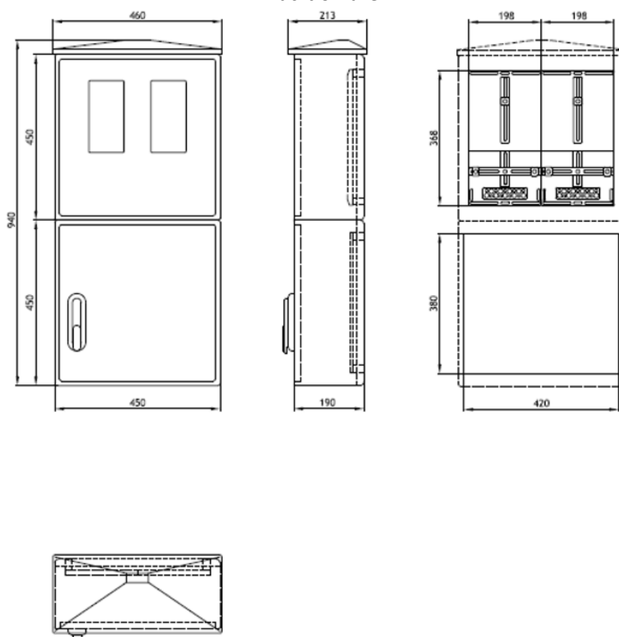
Načrt omare
