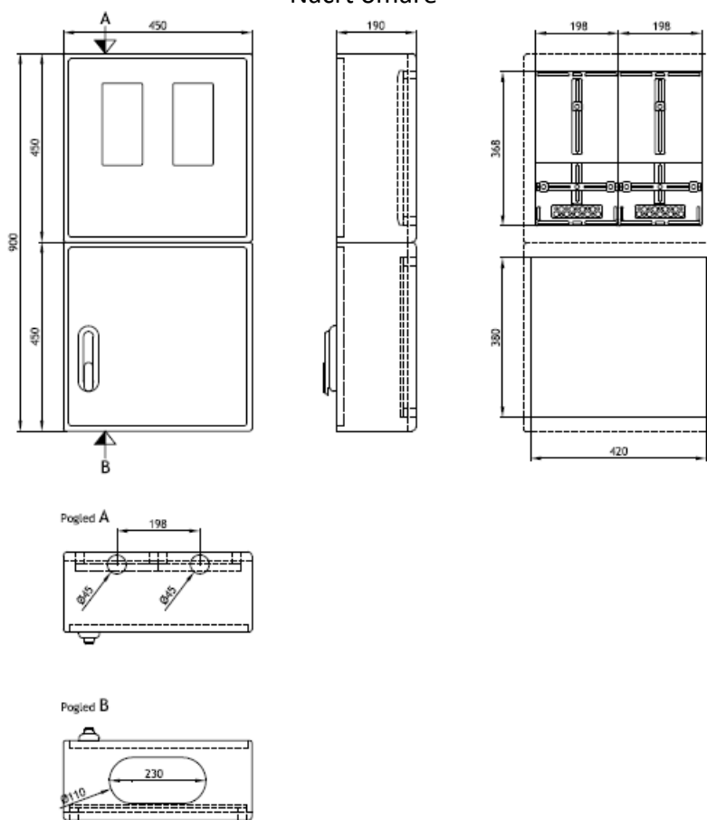
Načrt omare
